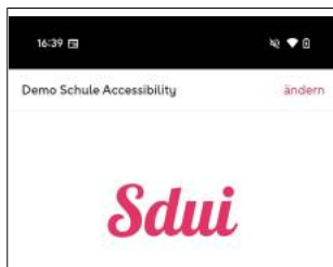
Ansicht 3 — Login
